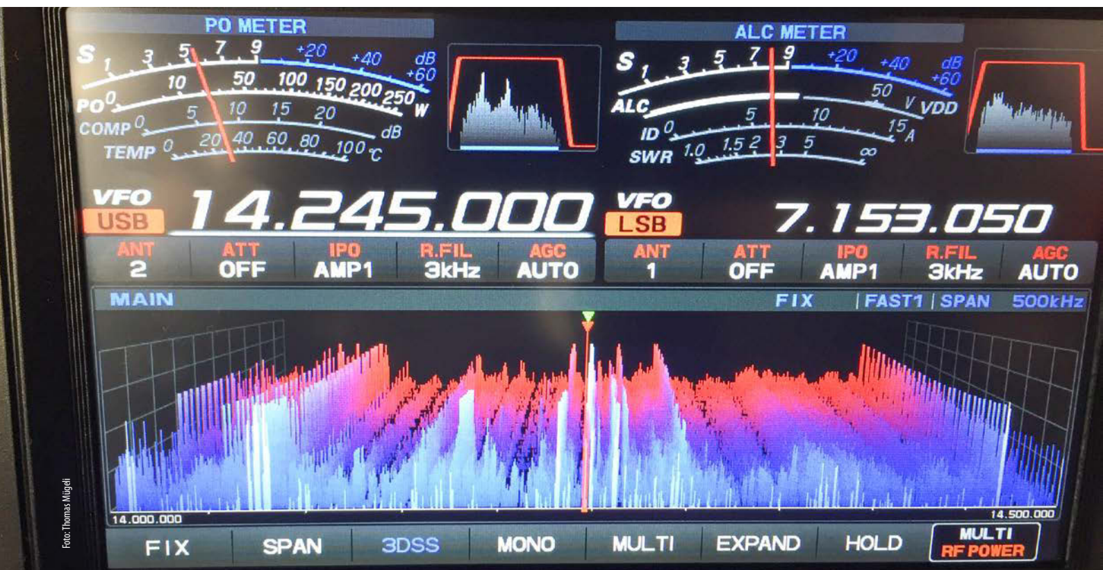
Typisches Störmuster durch DC-Optimierer im 20-Meter-Band (14 Megahertz) eines Amateurfunkers.
