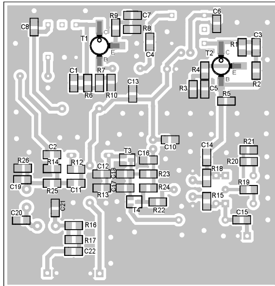
Bestückung Unterseite
